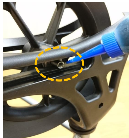
取り付け図
