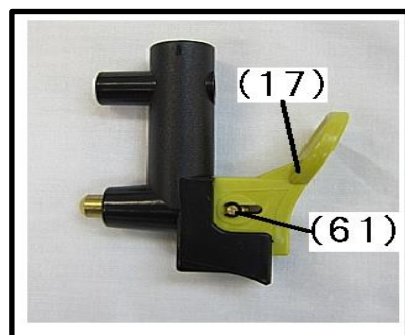
拡大図：(No16はNo.17.No.61と組んだ状態です)
