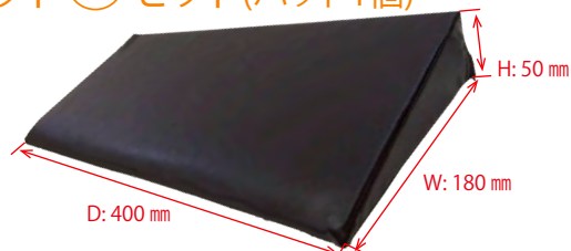
パッド⑤セット(パッド1個)
